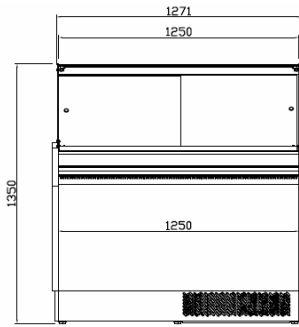
ALZADO
